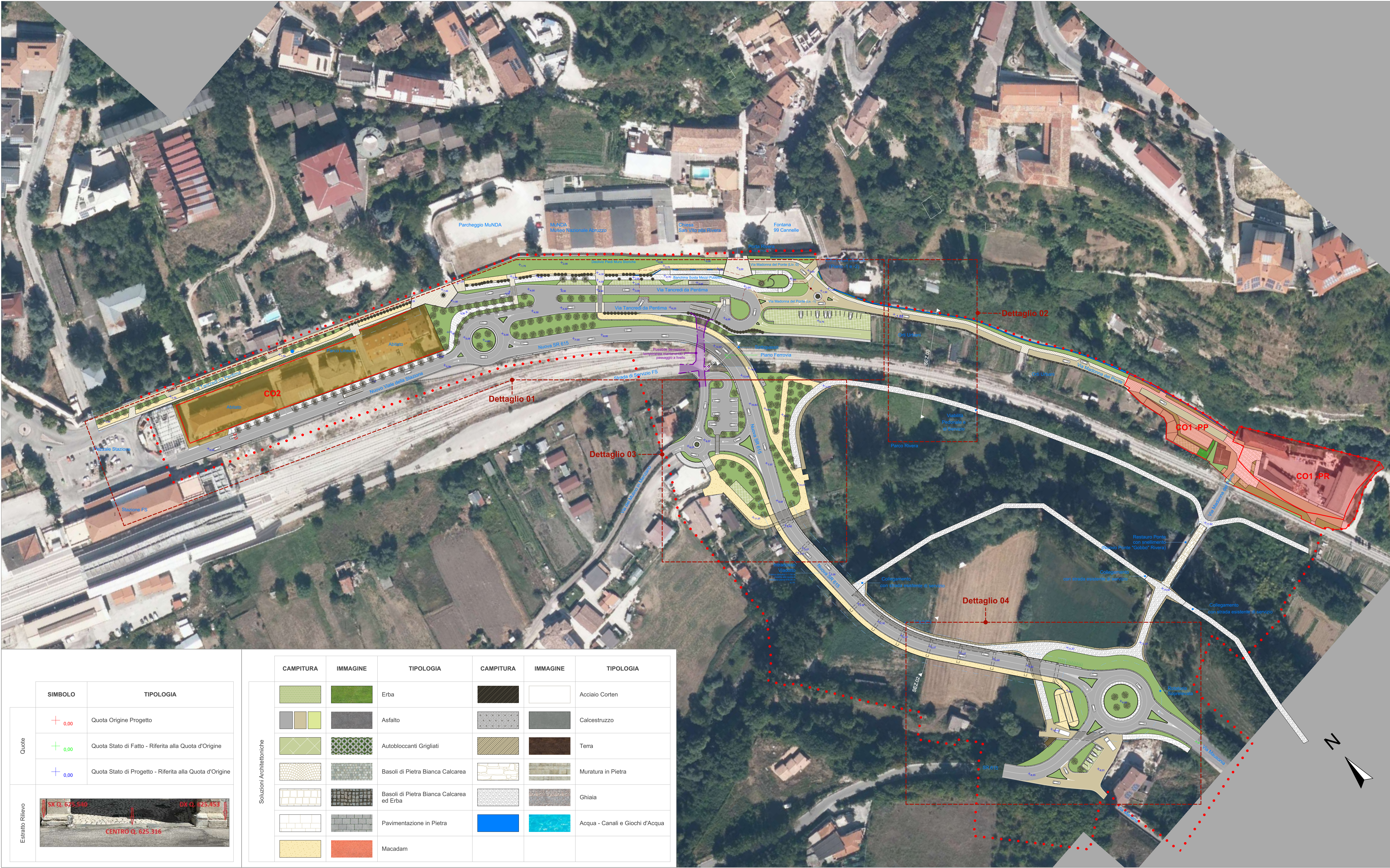
1:1000 Planimetria Generale
