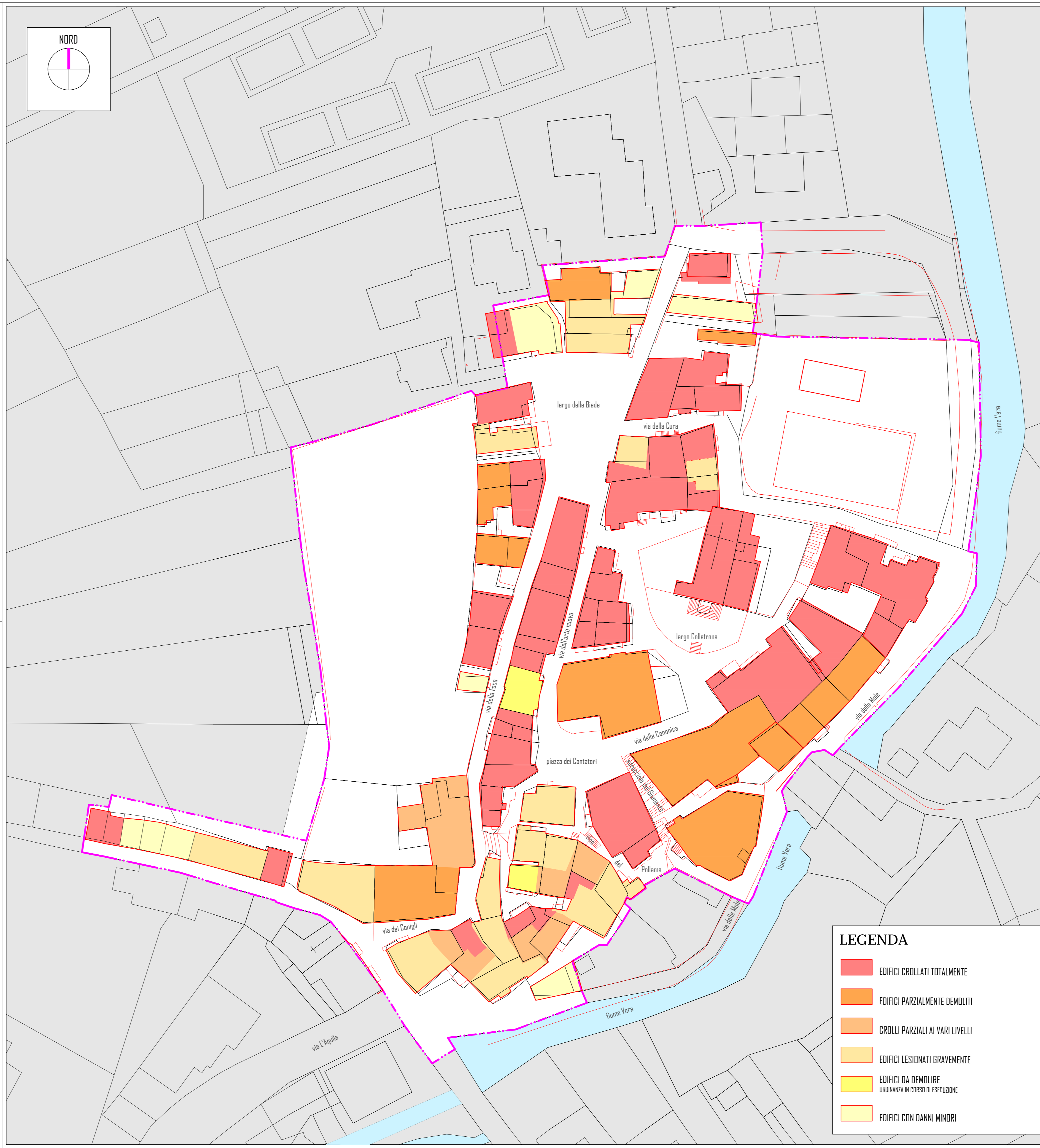
INDIVIDUAZIONE DEI DANNI E DEI CROLLI PLANIMETRIA GENERALE
